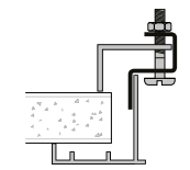
F5 - Patilha para Pladur
