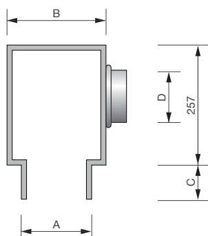
Fixação por patilha
