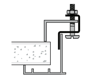
F5 - Patilha para Pladur
