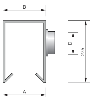
Fixação por ponte de montagem
