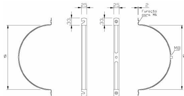
Desenho técnico de abraçadeiras com diâmetro até 300mm.
